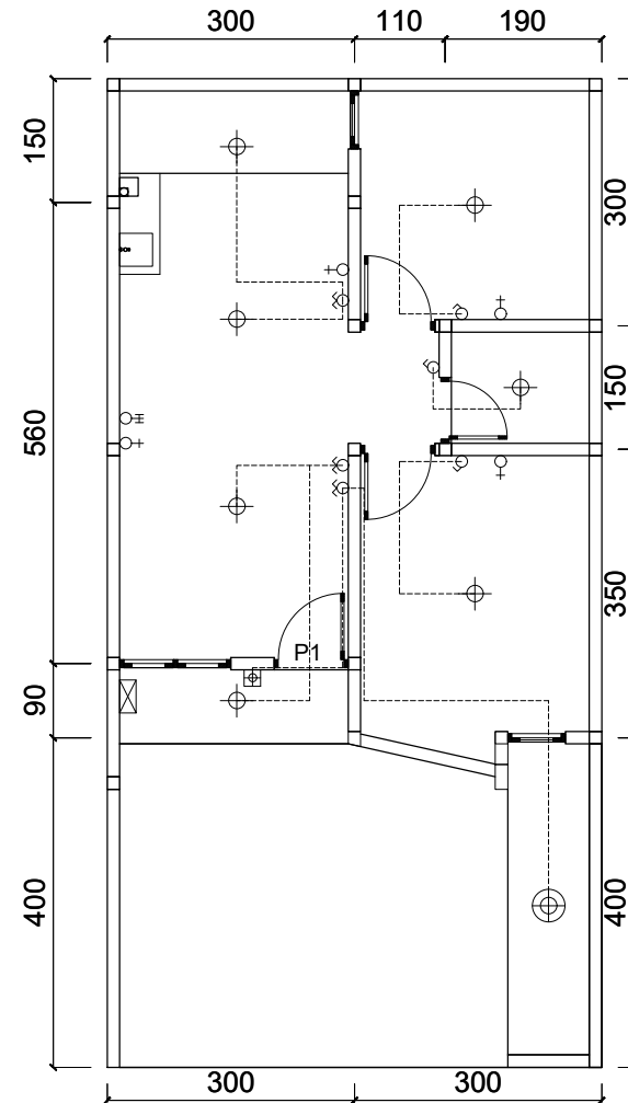
RENCANA LISTRIK
