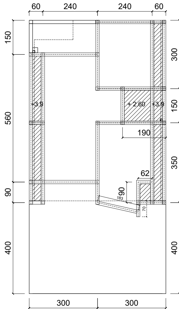
RENCANA ATAP
