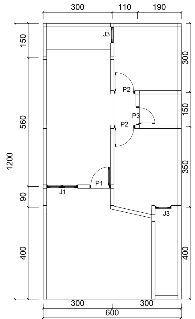
RENCANA KUSEN
