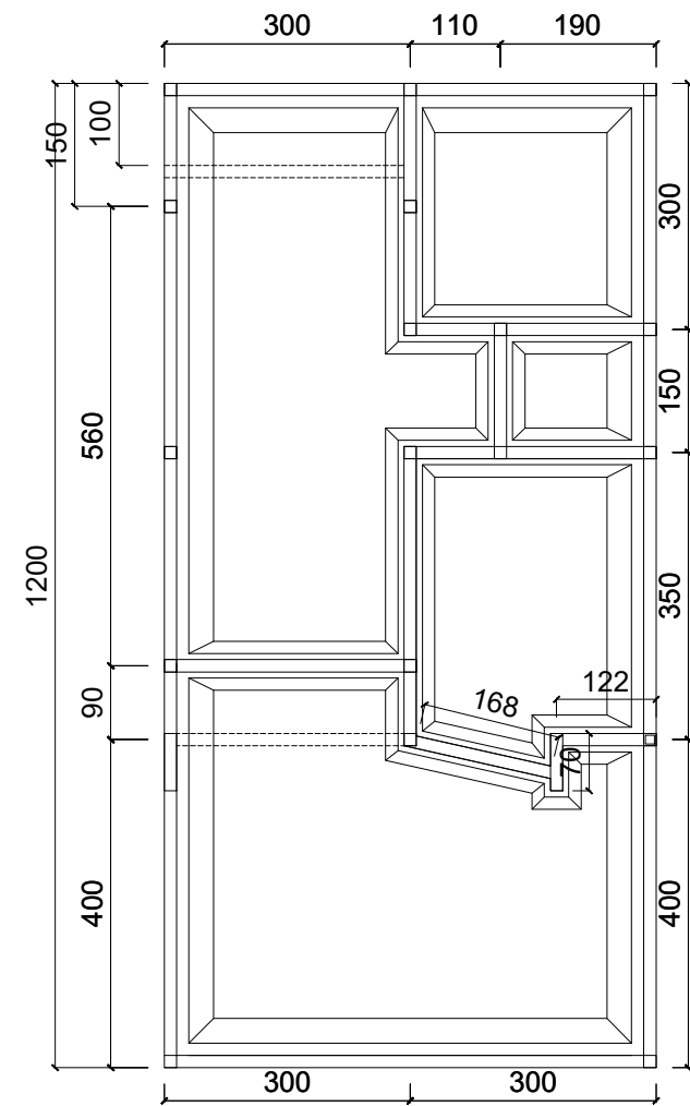
RENCANA PONDASI
