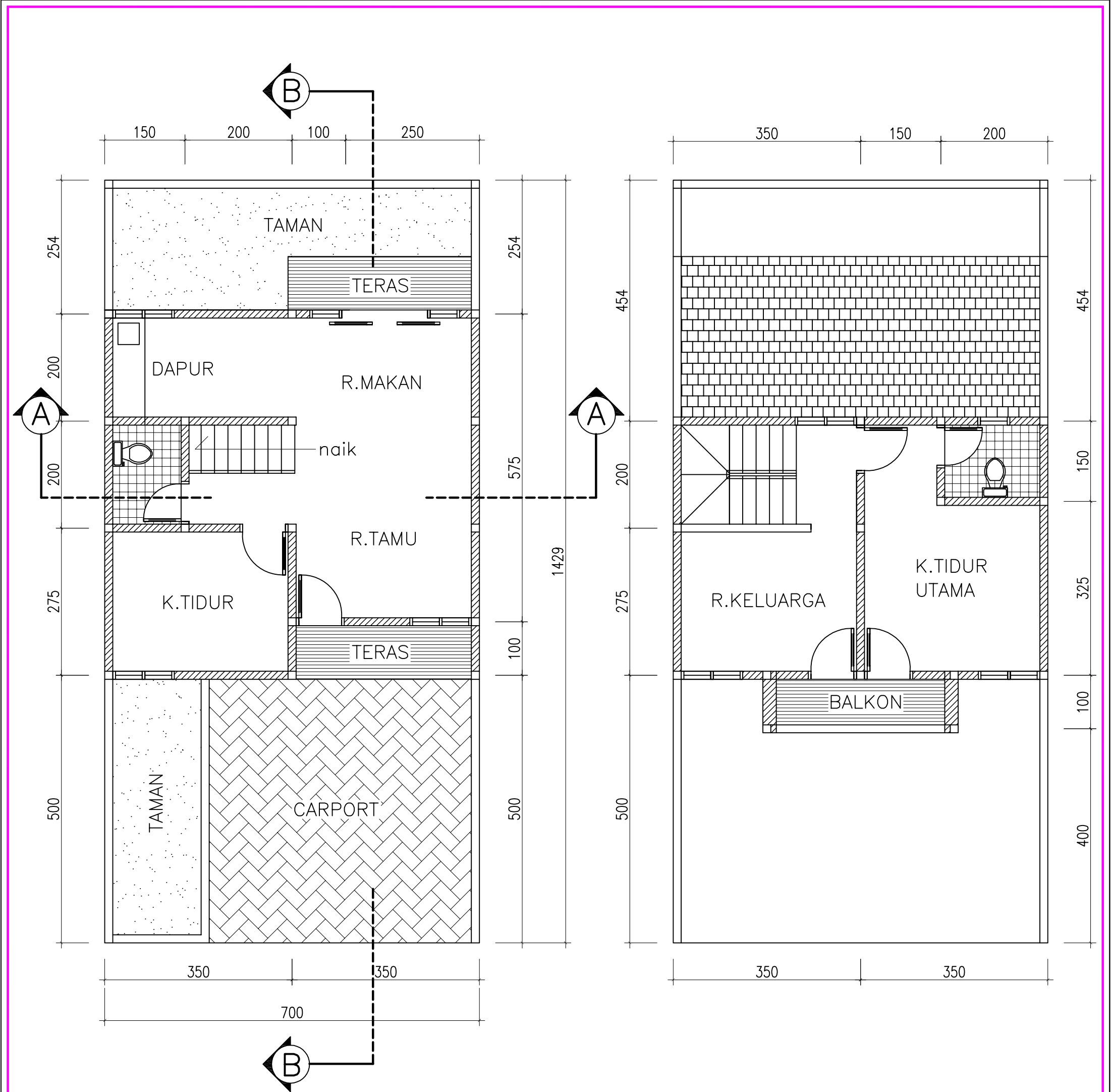
DENAH LT.BAWAH
