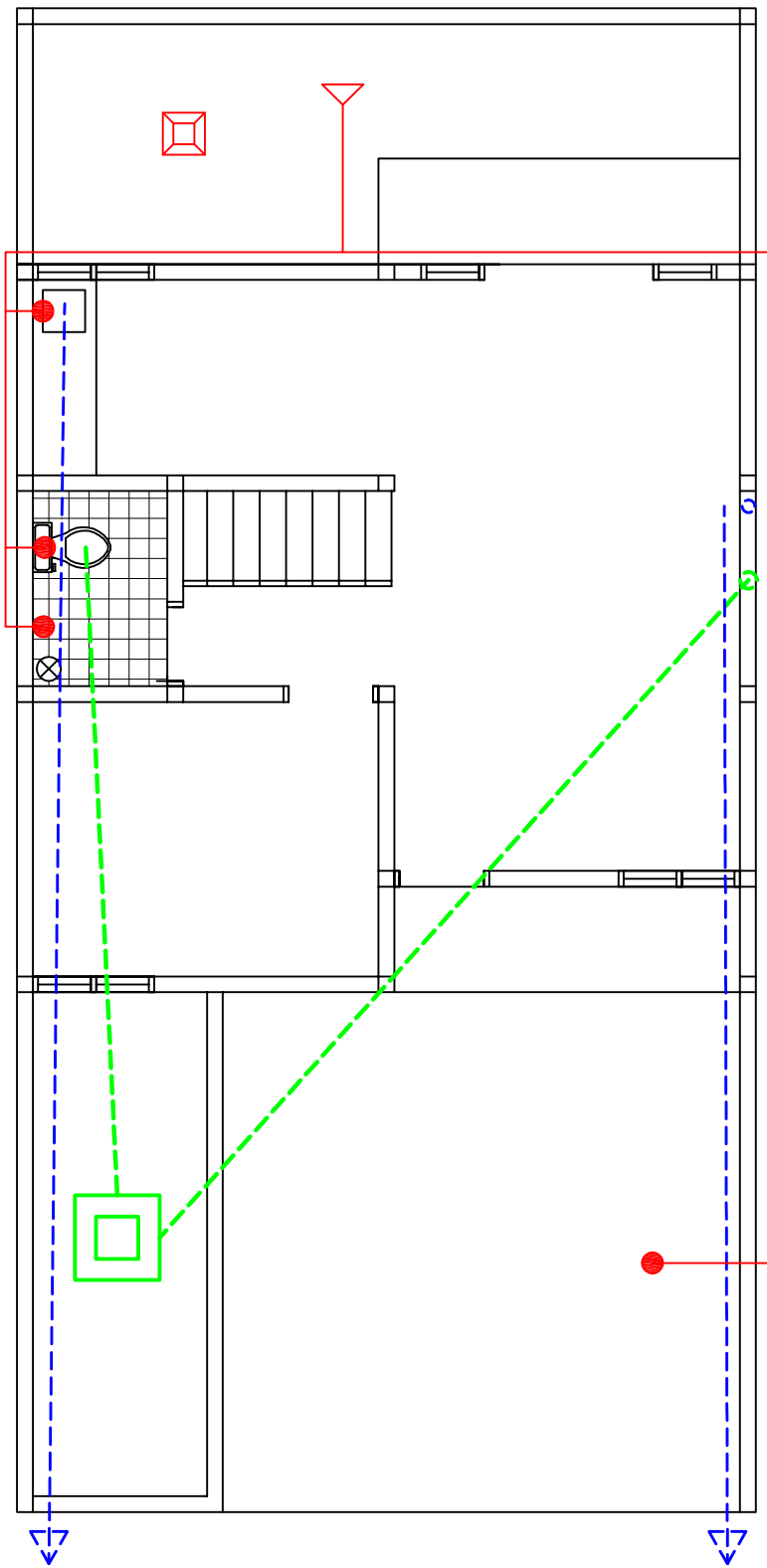
DENAH LT.BAWAH
